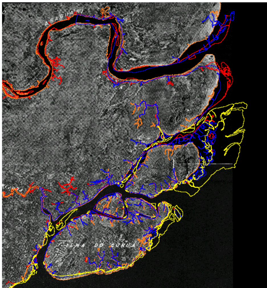
Figura 06: Modificações ocorridas durante os últimos 27 anos na região. A linha laranja mostra a configuração da linha de costa em 1974; a azul , em 1997; a vermelha em 2000, a amarela representa a acreção de bancos, registrada na imagem do ano de 2000.
