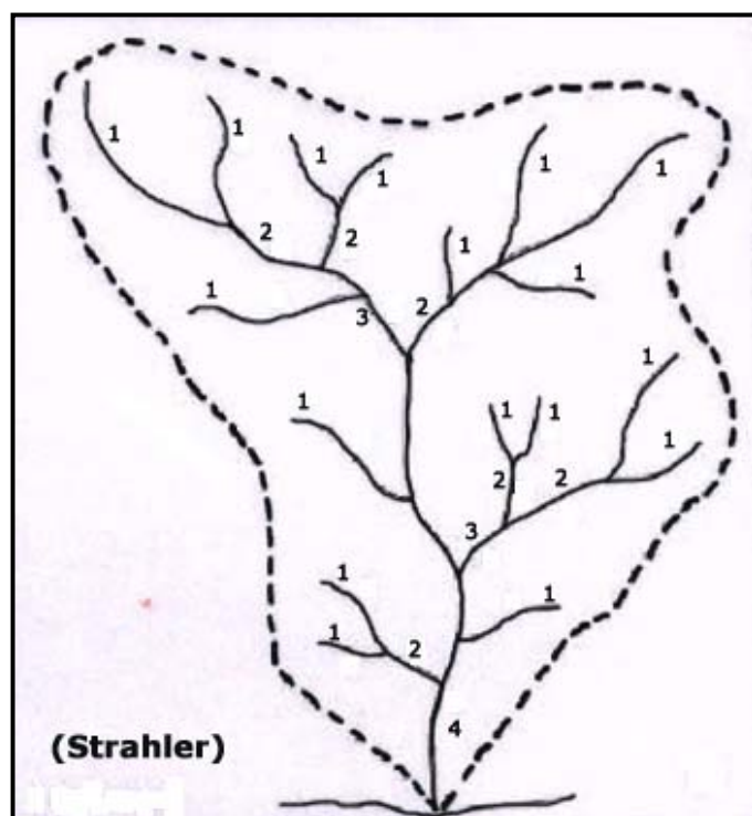
Figura 02: Modelo de hierarquização de bacia, proposto por Stralher (1952). Fonte: Lima (2002)
